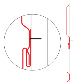
VERTIKALNA MONTAŽA
