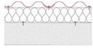
FASADNO PROFILISANJE PRESEK VERTIKALNE MONTAŽE
